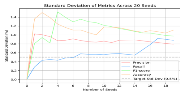
نمودار ۲: انحراف معیارهای ارزیابی مدل class weighting در ۲۰ seed نمودار ۳: انحراف معیارهای ارزیابی مدل k-fold cross-validation در ۲۰ seed
