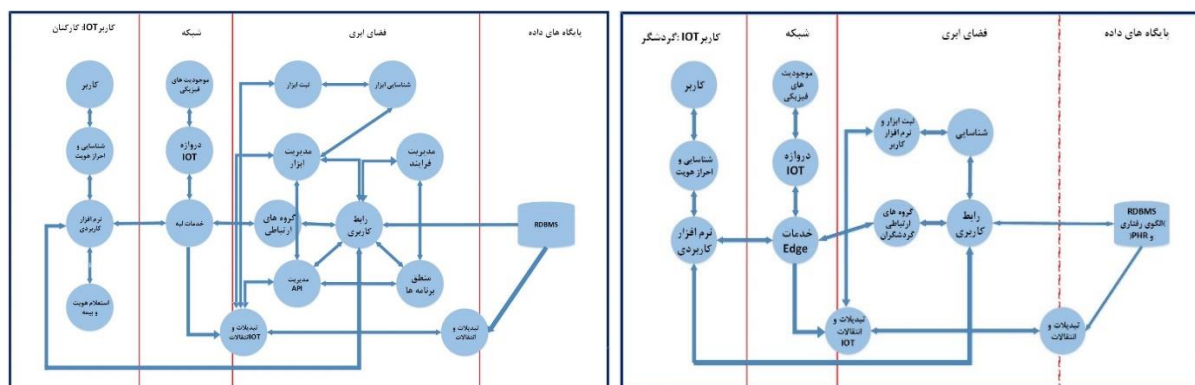
شکل ۱: معماری سرویس‌گرا
