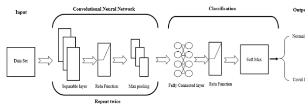
شکل ۳: معماری شبکه یادگیری عمیق
