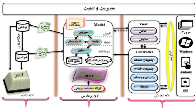
شکل ۳: مدل پیشنهادی معماری نرم‌افزار برای سیستم‌های CIS با استفاده از سبک طراحی MVC
