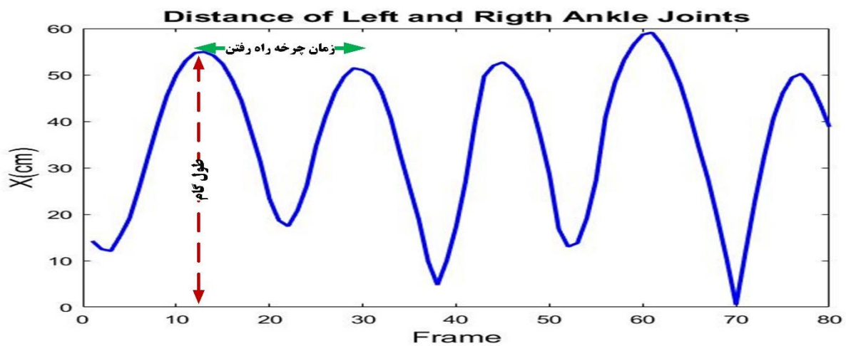
ب. ویژگی‌های راه رفتن از روی سیگنال فاصله مچ پاهای راست و چپ شکل ۶: یافتن ماکزیمم‌ها در سیگنال فاصله مچ پاها و استخراج ویژگی‌ها
