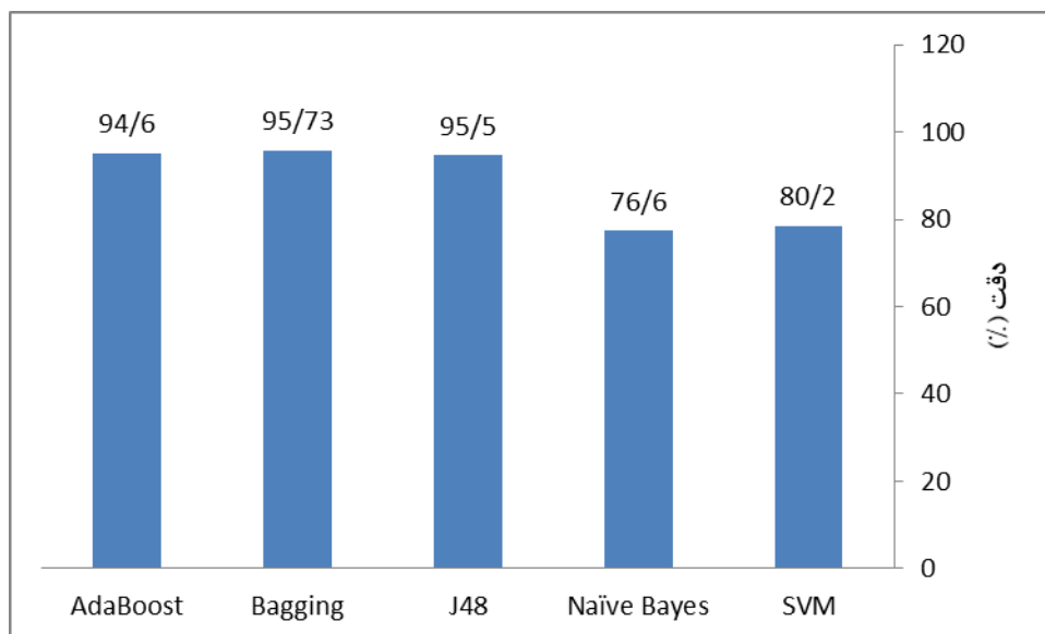
شکل ۲: مقایسه دقت الگوریتم‌های طبقه‌بندی
