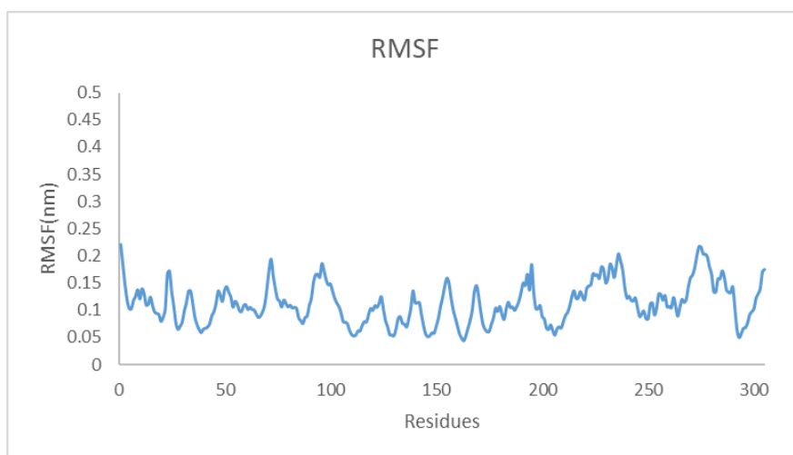
شکل ۴: نمودار RMSF برای کمپلکس cyanidin-3 5-di-o-glucoside و M pro
