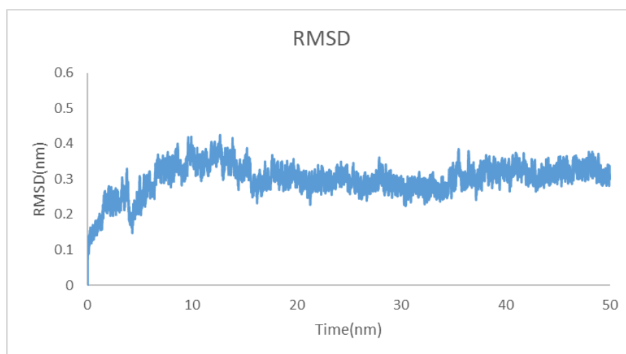
شکل ۳: نمودار RMSD برای کمپلکس cyanidin-3 5-di-o-glucoside و M pro
