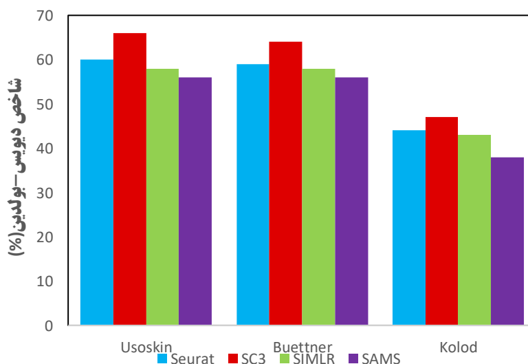
شکل ۳: مقایسه شاخص دیویس-بولدین روش‌های مختلف با روش پیشنهادی SAMS
