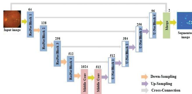
شکل ۳: ساختار شبکه Unet
