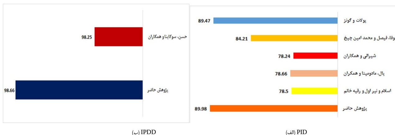
شکل ۱۳: مقایسه روش‌های مختلف پیاده‌سازی شده برای پیش‌بینی بیماری دیابت از نظر دقت طبقه‌بندی
