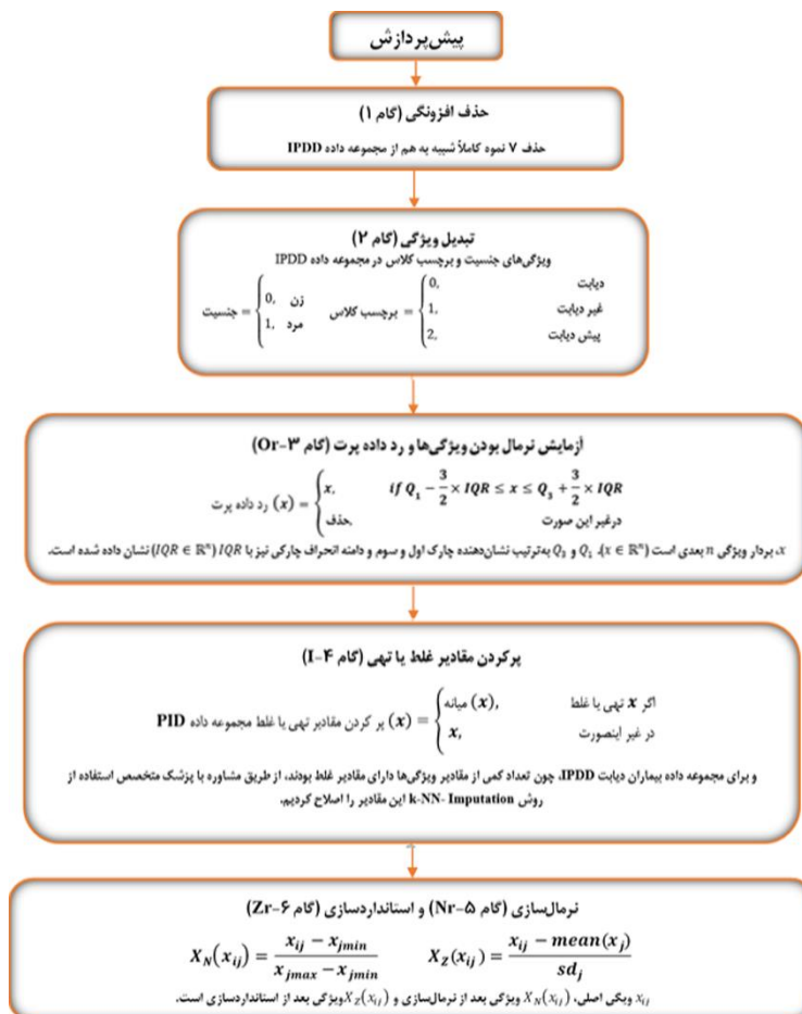
شکل ۲: گام‌های پیش پردازش
