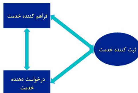
شکل ۱: معماری سرویس‌گرا
