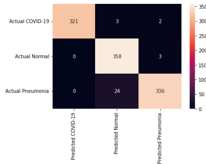
الف) EfficientNet-B4 network
