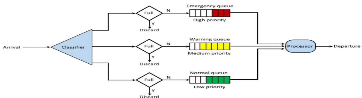
شکل ۲: طبقه‌بندی درخواست‌ها در صف‌های اولویت لایه مه
