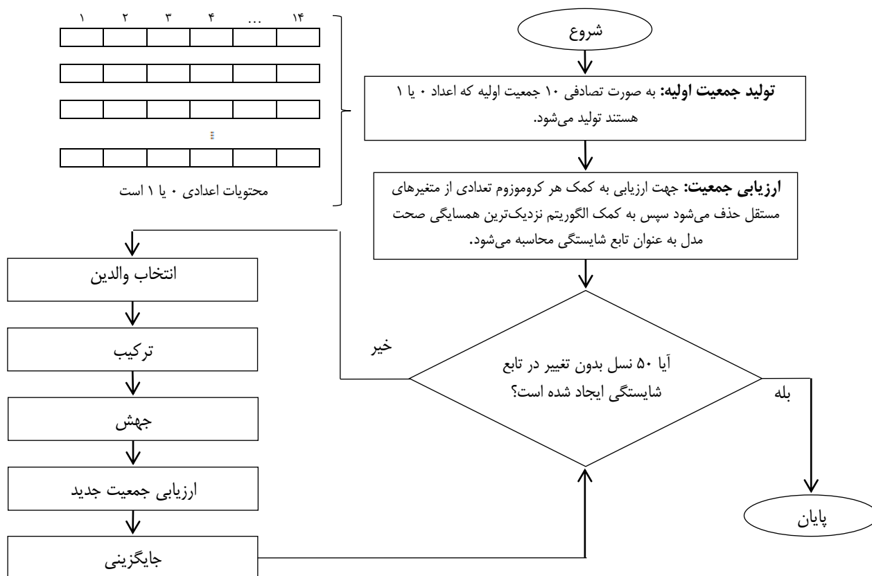
شکل ۶: الگوریتم ژنتیک پیشنهادی برای کاهش تعداد متغیرها مستقل
