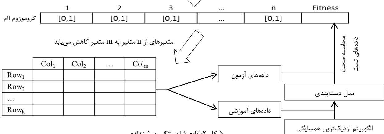
شکل ۲: تابع شایستگی پیشنهادی
