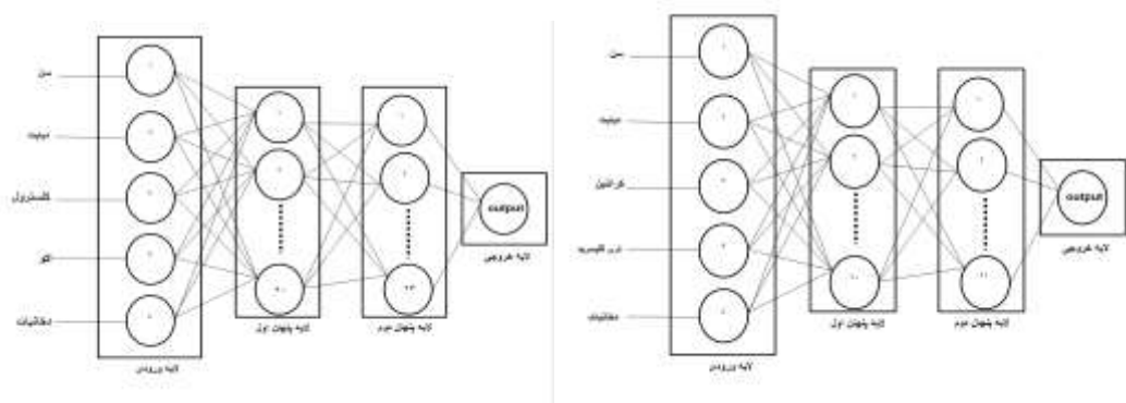
شکل ۲-۳ طراحی شبکه عصبی N3 با ورودی‌های
